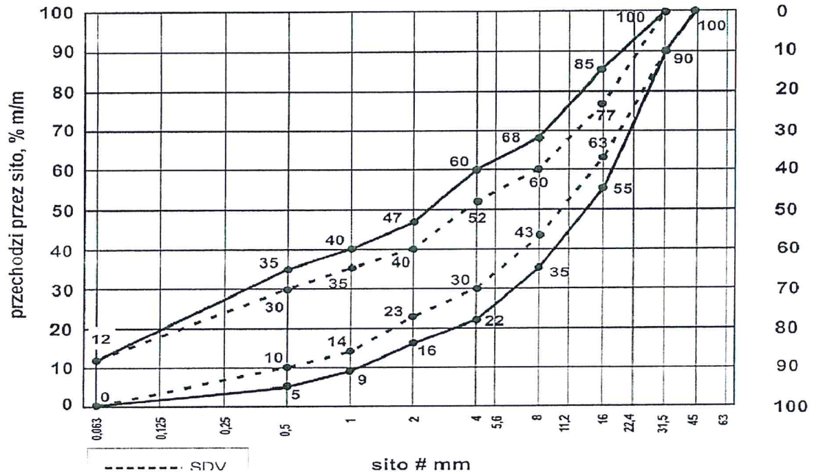
Rys. 2. Mieszanka niezwiązana 0/31,5 do warstw podbudowy zasadniczej
